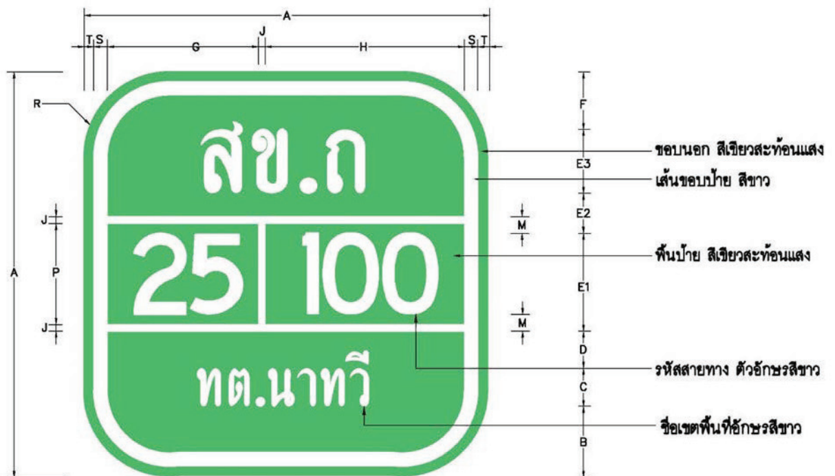
รูปที่ ข-๗ ตัวอย่างและรายละเอียดป้ายหมายเลขทางหลวงท้องถิ่น (น-๑/๑) ขนาด ๗๕x๗๕ ซม. (สำหรับ อปท. ลำดับที่ ๑๐ - ๙๙)
