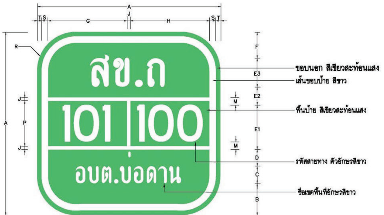
รูปที่ ข-๙ ตัวอย่างและรายละเอียดป้ายหมายเลขทางหลวงท้องถิ่น (น-๑/๑) ขนาด ๗๕x๗๕ ซม. (สำหรับ อปท. ลำดับที่ ๑๐๐- ๙๙๙)
