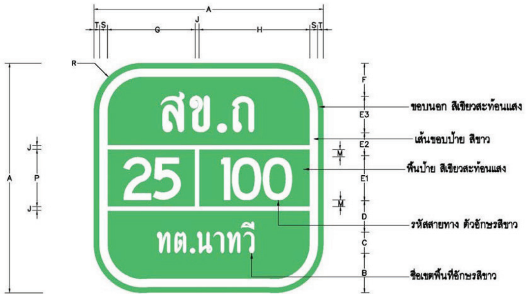
รูปที่ ข-๖ ตัวอย่างและรายละเอียดป้ายหมายเลขทางหลวงท้องถิ่น (น-๑/๑) ขนาด ๖๐x๖๐ ซม. (สำหรับ อปท. ลำดับที่ ๑๐ - ๙๙)
