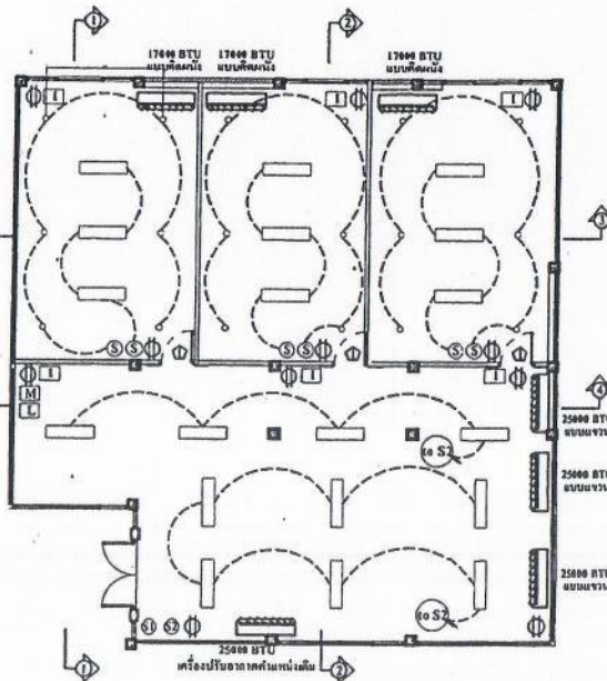
ผังไฟฟ้าหลังปรับปรุง มาตราส่วน 1 : 150
