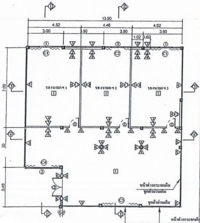
ผังพื้นที่หลังปรับปรุง มาตราส่วน 1 : 150
