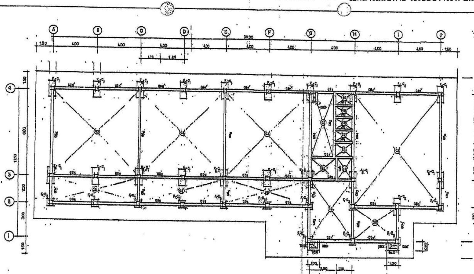
แบบฐานราก-คานคอดิน
