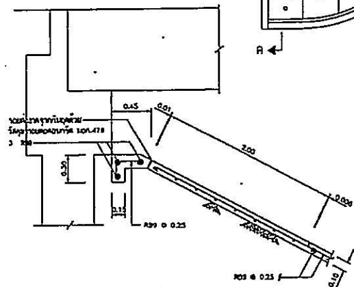
แบบขยาย 1 ขนาดหน้า 1 : 25
