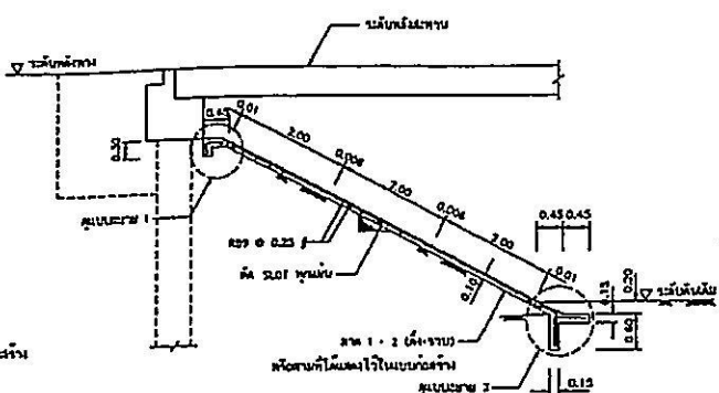
รูปตัด ก - ก ขนาดหน้า 1 : 50
