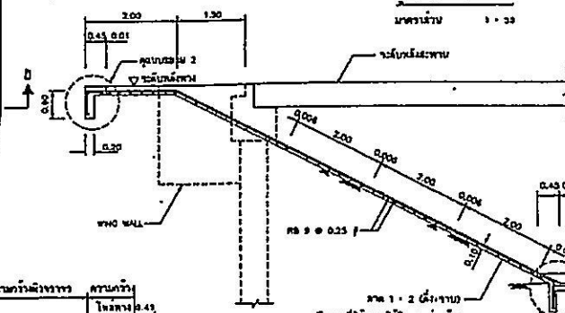
รูปตัด ข - ข ขนาดหน้า 1 : 50
