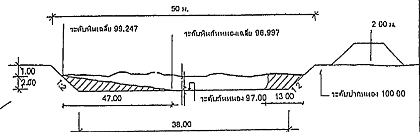
รูปตัด A — A
