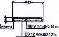
แบบขยายฝาครอบ ค.ล.ล. มาตราส่วน 1 : 30
