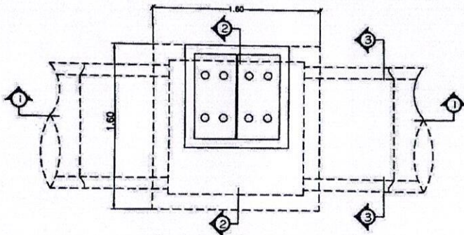
แปลนท่อระบายน้ำขนาด ๑.๐๐x๑.๐๐ ม. scale 1 : 30
