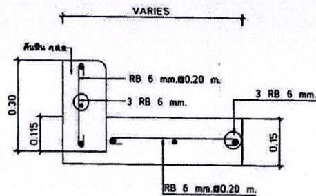
แบบขยายรางดิน มาตราส่วน 1 : 10
