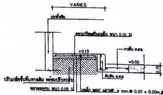
แบบขยายทางเท้า มาตราส่วน 1 : 25
