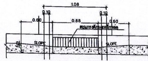
รูปด้านหน้า ช่องระบายน้ำ มาตราส่วน 1 : 25
