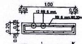
ขยาย ช่องระบายน้ำ มาตราส่วน 1 : 25
