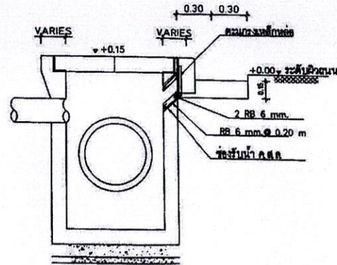
รูปตัดช่องรับน้ำจากผิวจราจรลงบ่อพัก มาตราส่วน 1 : 25
