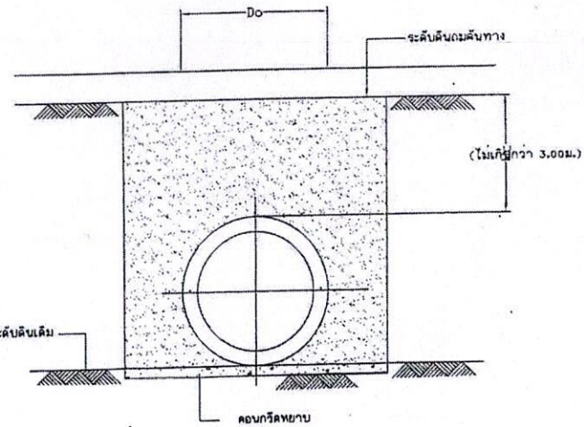
กรณีแควงเดียว
