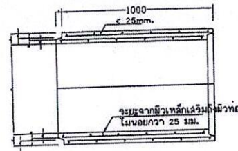
รูปตัดตามยาวแสดงรายละเอียดท่อระบายน้ำ ค.ฉ.ค.แบบปากลิ้นราง
