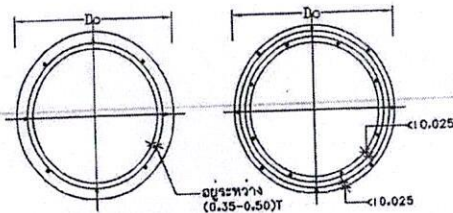
ฉ. รูปตัดขวางแสดงการเสริมเหล็กขึ้นด้วยแควงและข้อ
