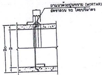
ข. รูปตัดแสดงการต่อท่อยาแนว
