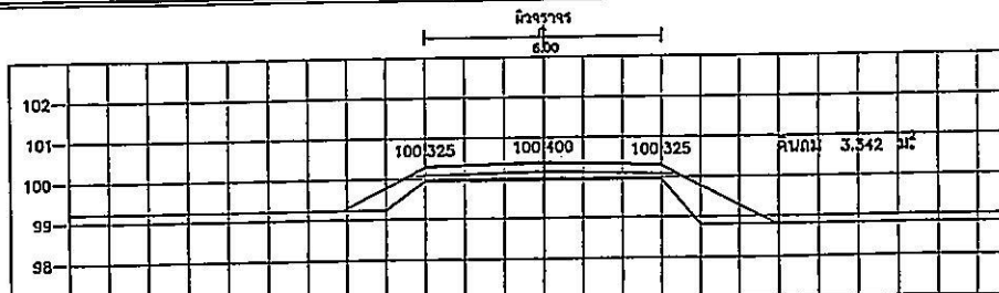
STA. 0+400.000 NGL = 99.946
