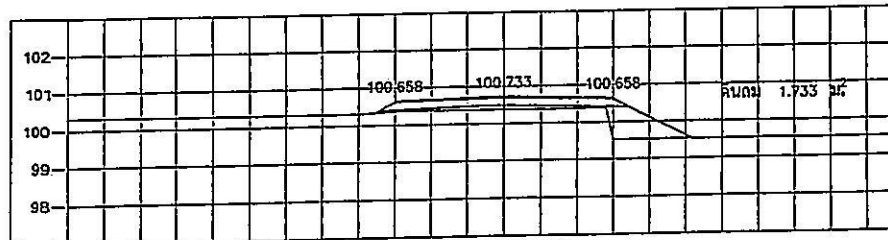
STA. 0+050.000 NGL = 100.380
