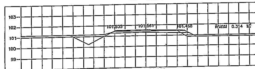
STA. 0+950.000 NGL = 101.450
