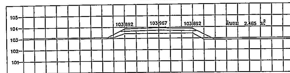
STA. 1+200.000 NGL = 103.444
