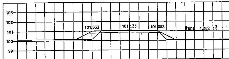
STA. 0+150.000 NGL = 101.040
