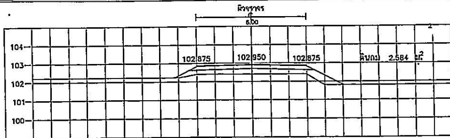
STA. 1+100.000 NGL = 102.402
