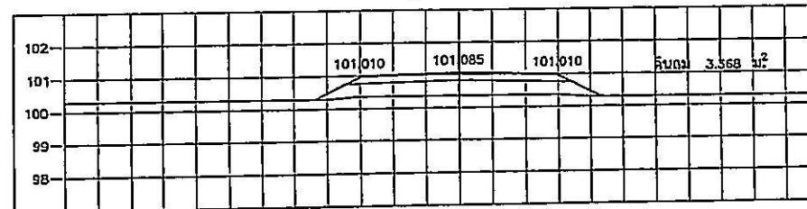
STA. 1+000.000 NGL = 100.372
