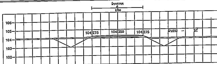
STA. 1+300.000 NGL = 104.170
