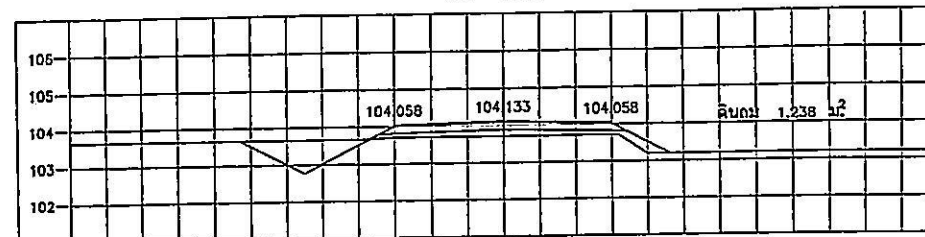
STA. 1+250.000 NGL = 103.712
