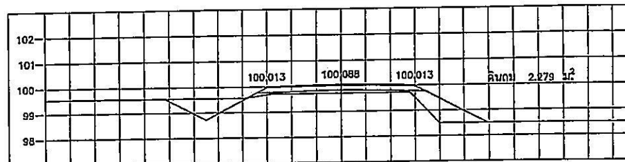
STA. 0+350.000 NGL = 99.716
