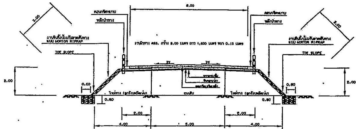
รูปตัด (ข) - (ช)
