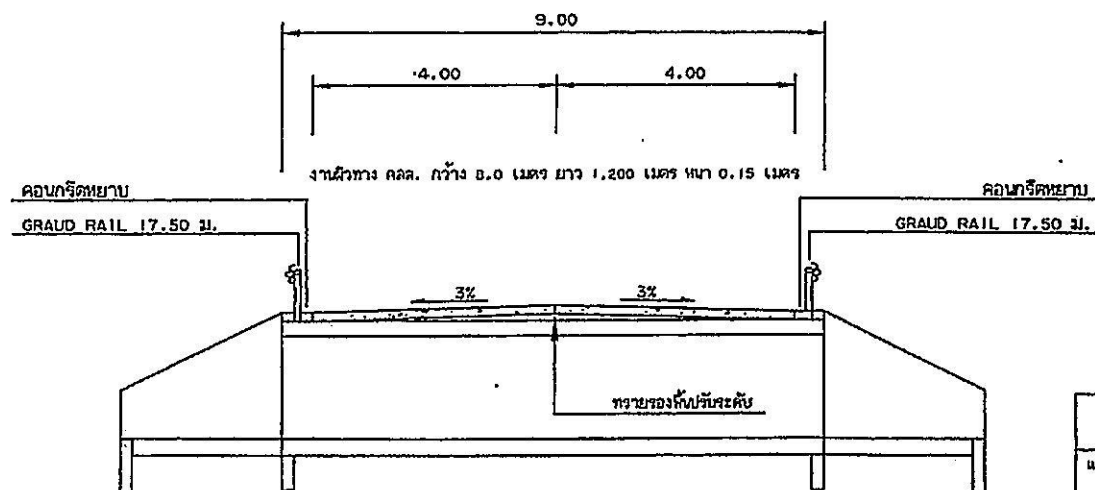
รูปตัด (ก) - (ก) ไม้คองมาทราถ่วน
