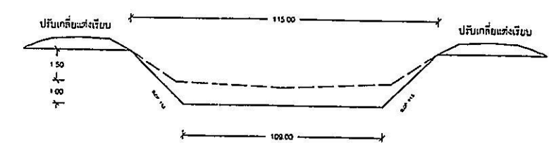
รูปตัด A - A มาตรฐาน ไม่ระบุ
