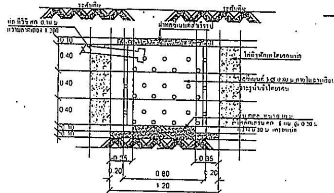
แบบขยายบ่อซึม มาตราส่วน NTS
