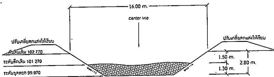
STA. 0+300
