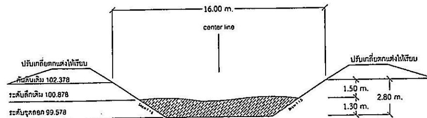
STA. 0+450
