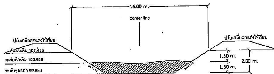
STA. 0+500
