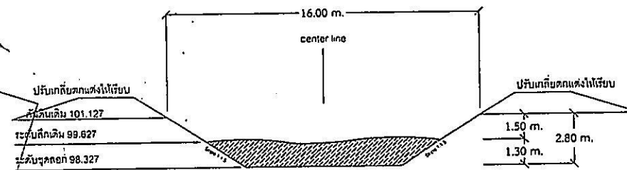
STA. 0+550
