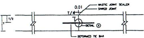
LONGITUDINAL JOINT
