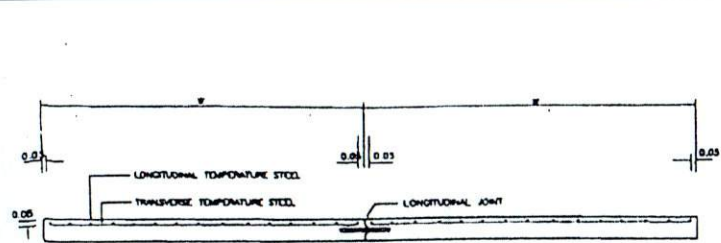
รูปตัดตามขวางผิวจราจร ค.ร.ร.
