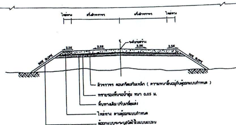
รูปตัดแสดงโครงสร้างถนนคอนกรีตเสริมเหล็กและคุณสมบัติวัสดุ ขนาดหน้า
