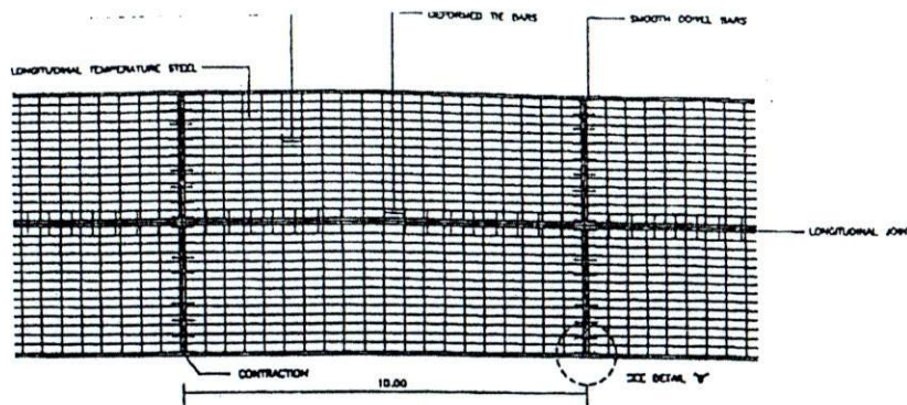
แบบแผนการเสริมเหล็กถนน ค.ร.ร.
