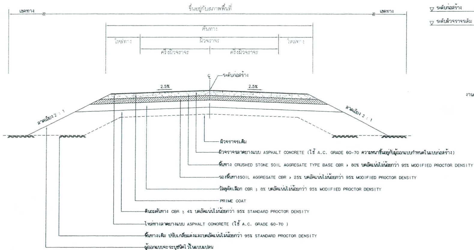
รูปตัดแฉดงโครงสร้างถนนและคุณสมบัติวัสดุ
