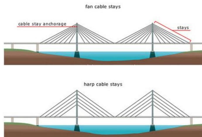
รูปภาพแสดงลักษณะของสะพานแบบฮาร์ป (harp) และแบบแฟน (fan)
