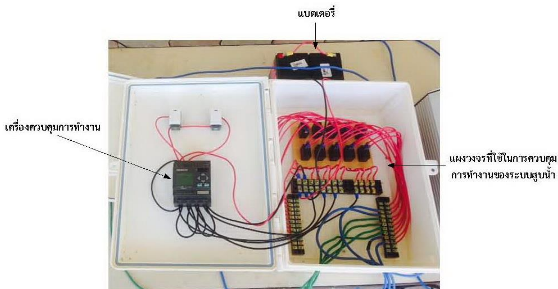
รูปภาพที่ 2 ระบบควบคุมทางไฟฟ้า
